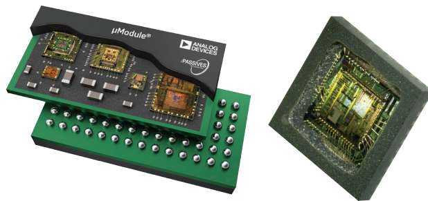
图3. 使用iPassives的 \mu Module产品示例。
