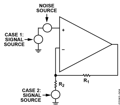
图5. 信号增益与噪声增益
