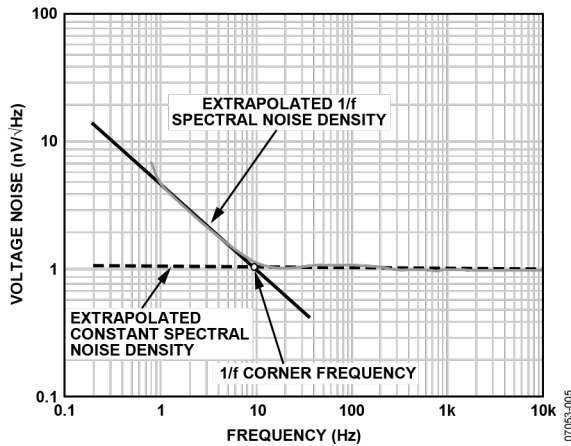
图2. 噪声谱密度
