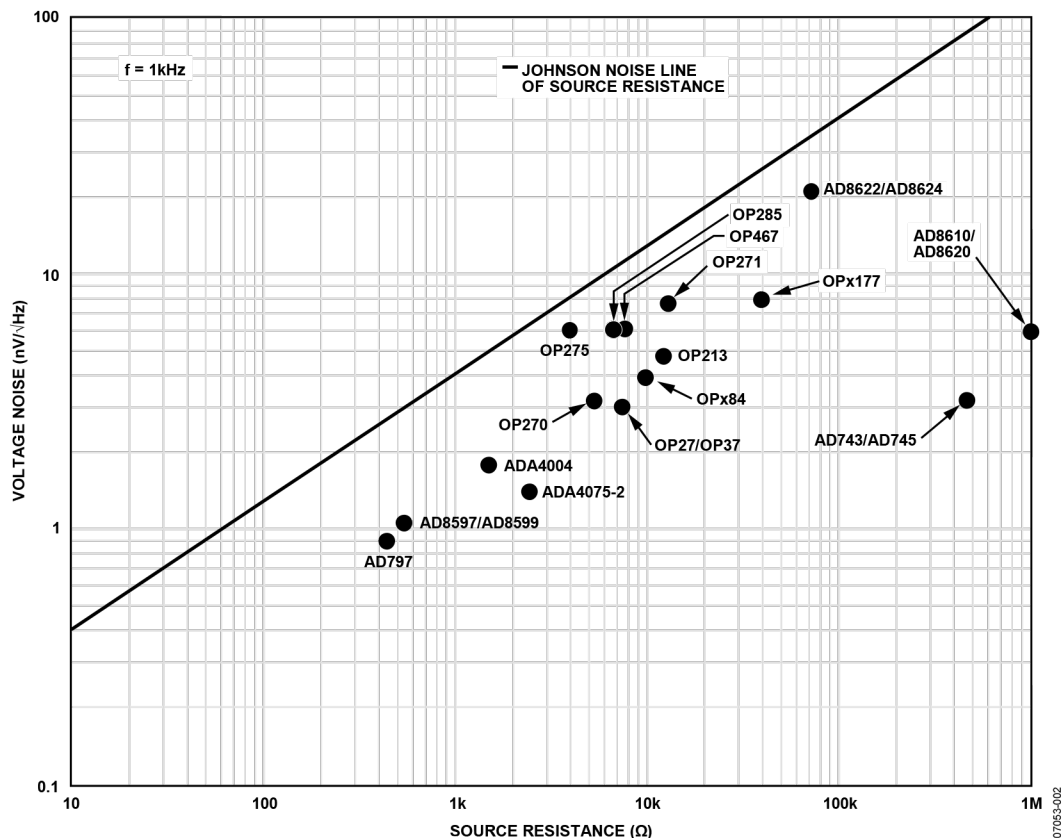
图6. ADI公司的运算放大器噪声图
