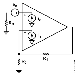
图1. 运算放大器噪声模型
