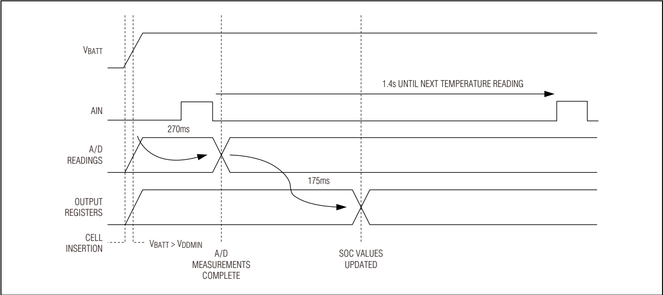
图37. 上电操作
