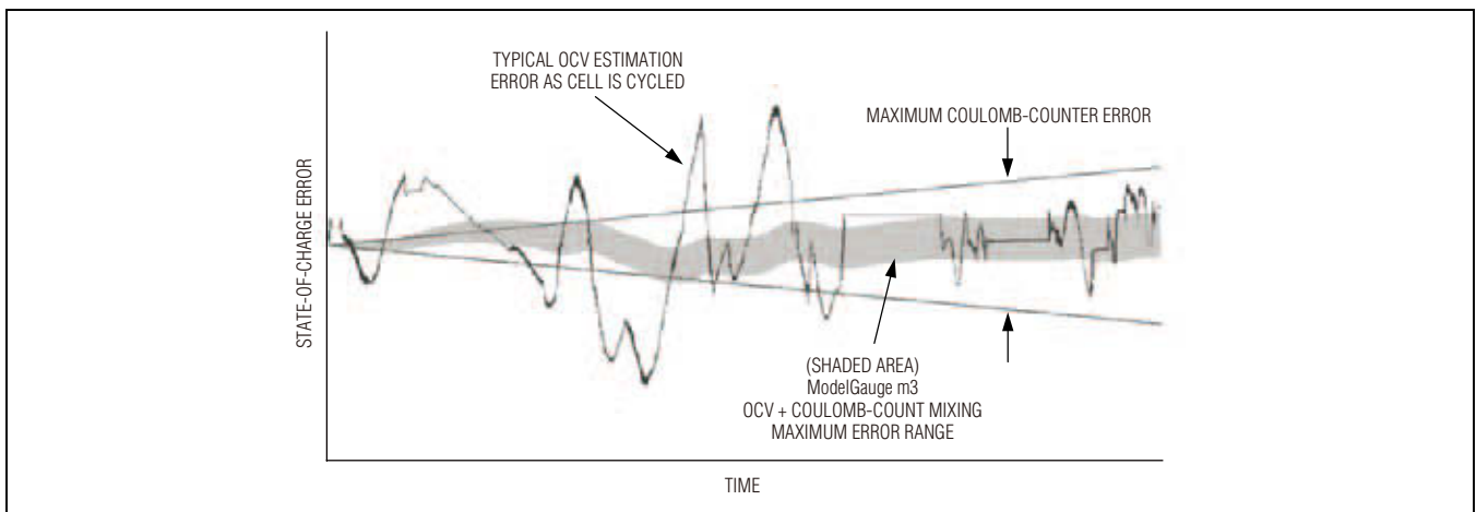
图4. ModelGauge m3混合算法原理示意图
