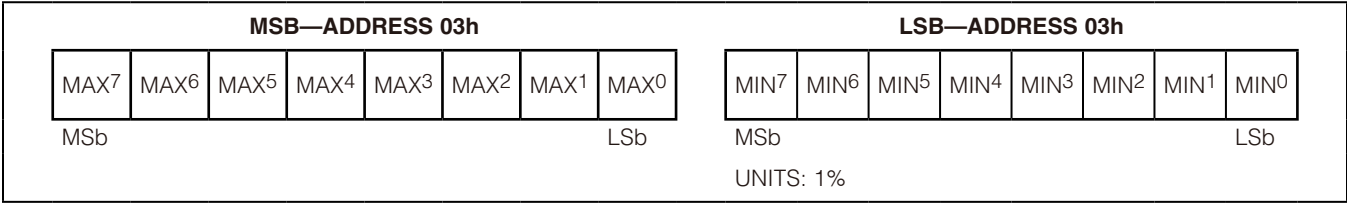
图43. S ALRT 门限寄存器格式(输入)
