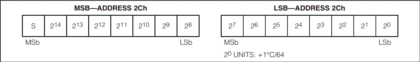
图61. TGAIN寄存器格式(输入)
