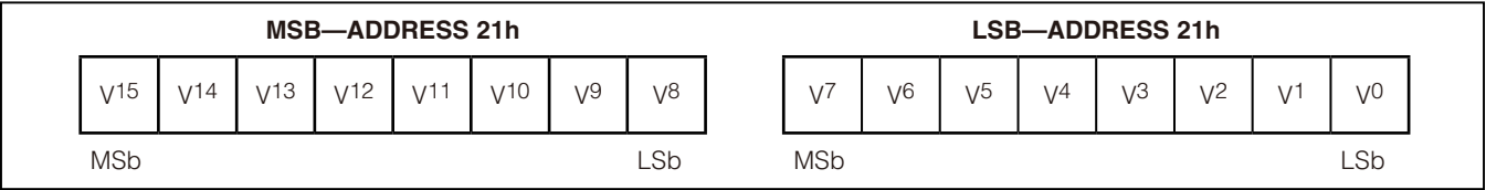
图48. 版本寄存器格式(输出)
