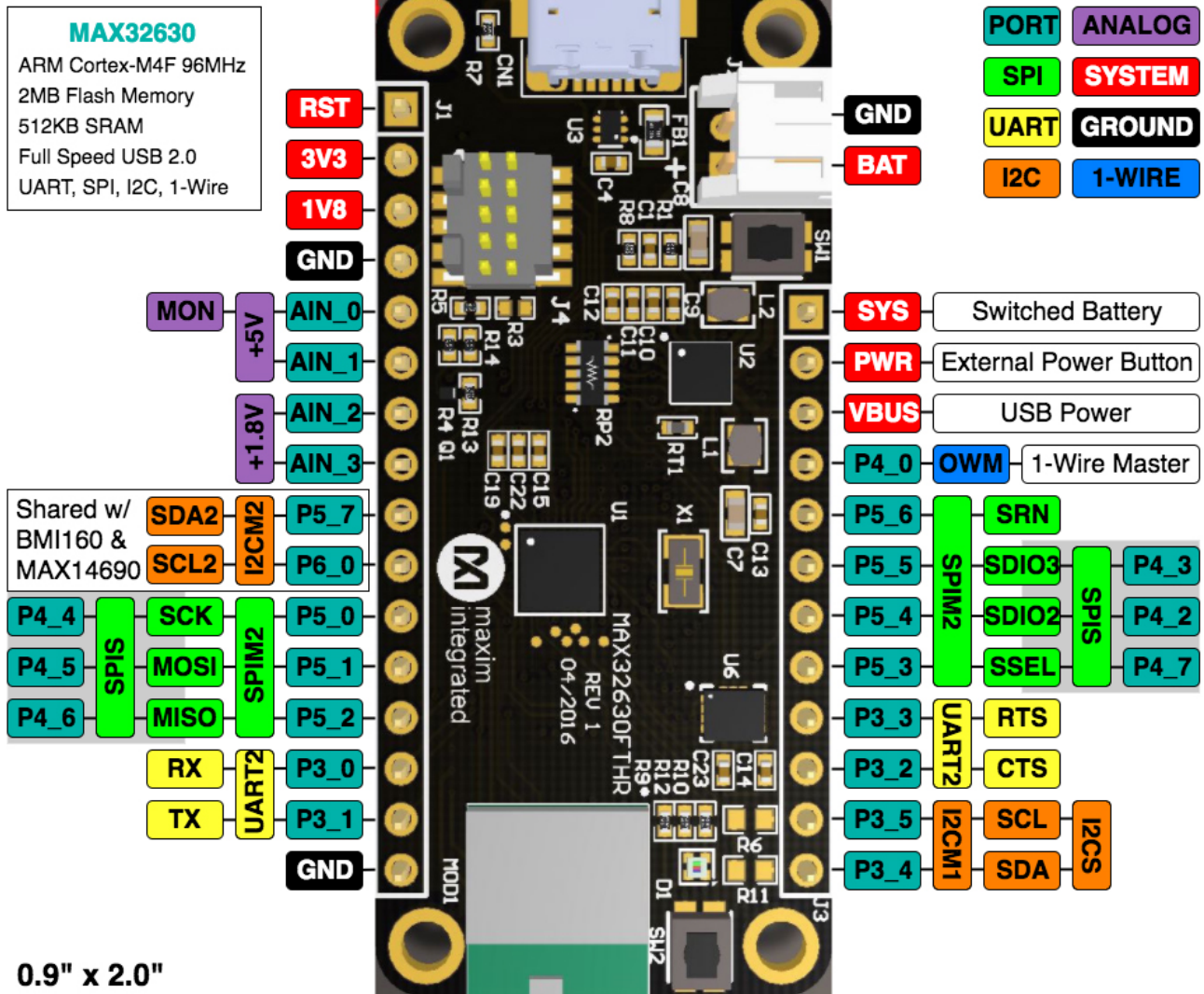
图1. MAX32630 FTHR引脚排列图
