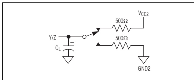
图3. 驱动器时序测试负载
