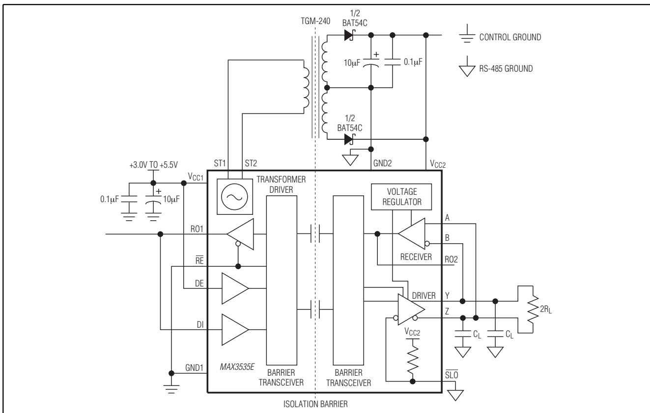
图5. 自激配置
