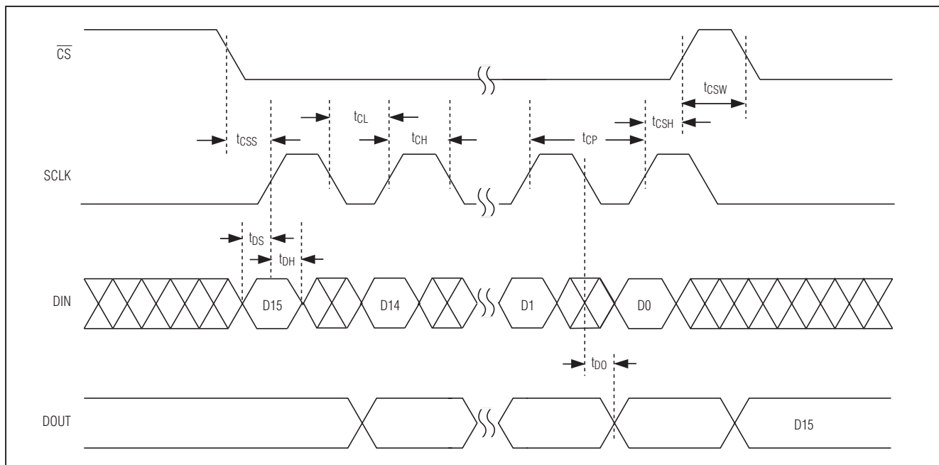
图4. 时序图
