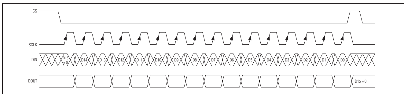
图5. 16位写操作发送至MAX7317
