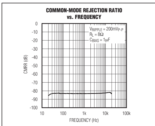
图3. 差分输入下的CMRR
