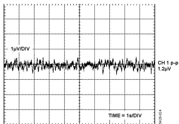
图28. ADR441 0.1 Hz至10.0 Hz电压噪声
