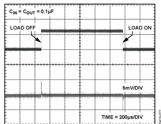
图27. ADR441负载瞬态响应
