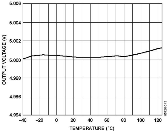
图9. ADR445输出电压与温度的关系
