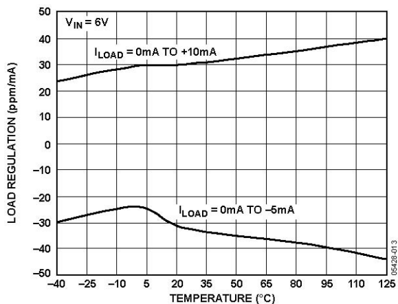
图17. ADR445 负载调整率与温度的关系
