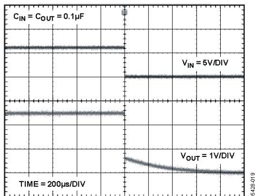
图23. ADR441关断响应
