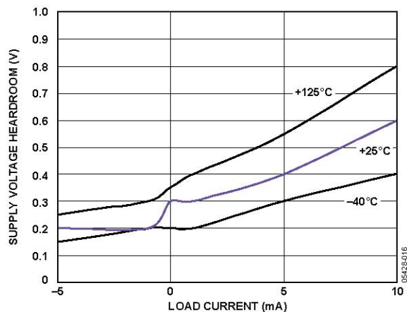
图20. ADR445 电源电压裕量与负载电流的关系
