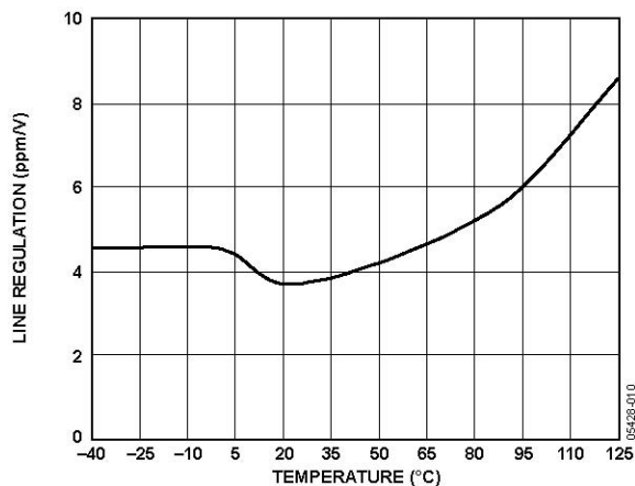
图14. ADR441电压调整率与温度的关系
