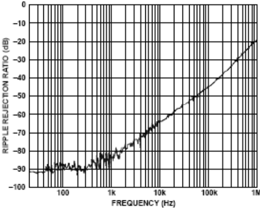
图34. 纹波抑制比与频率的关系
