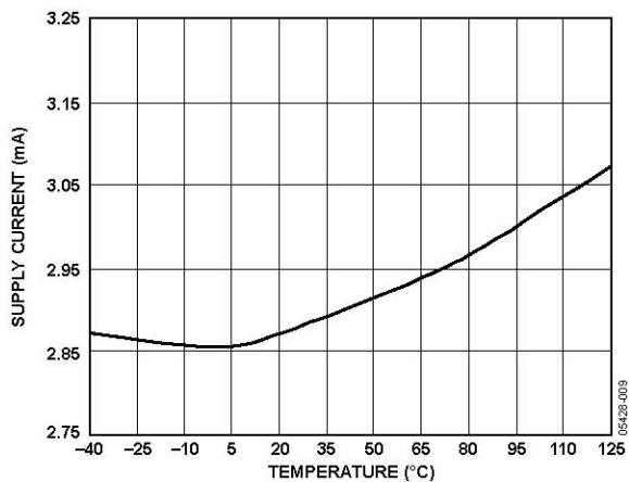
图13. ADR445电源电流与温度的关系
