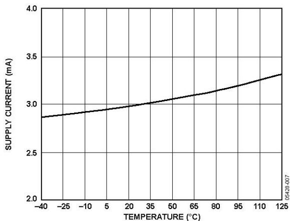
图11. ADR441电源电流与温度的关系
