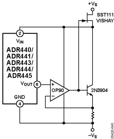
图41. 浮动电流源
