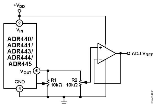
图39. 可编程电压源
