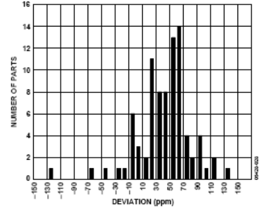
图32. ADR441 典型输出电压迟滞
