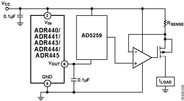
图40. 可编程电流源
