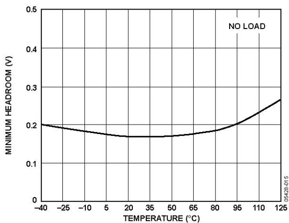
图19. ADR441 最小裕量与温度的关系
