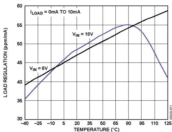
图15. ADR441负载调整率与温度的关系
