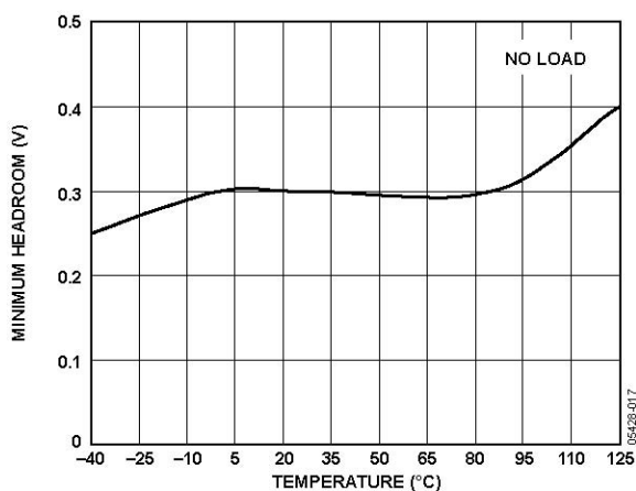
图21. ADR445 最小裕量与温度的关系
