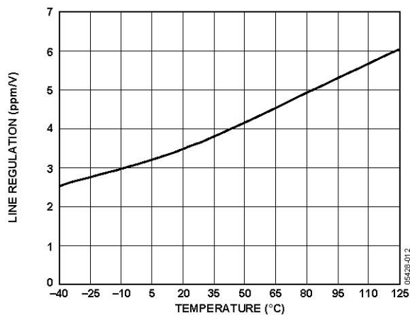
图16. ADR445电压调整率与温度的关系
