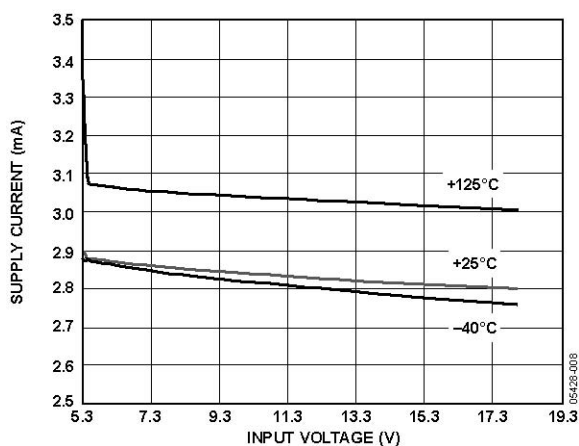
图12. ADR445电源电流与输入电压的关系
