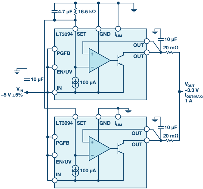
图 3. 两个并联 LT3094 的原理图。
