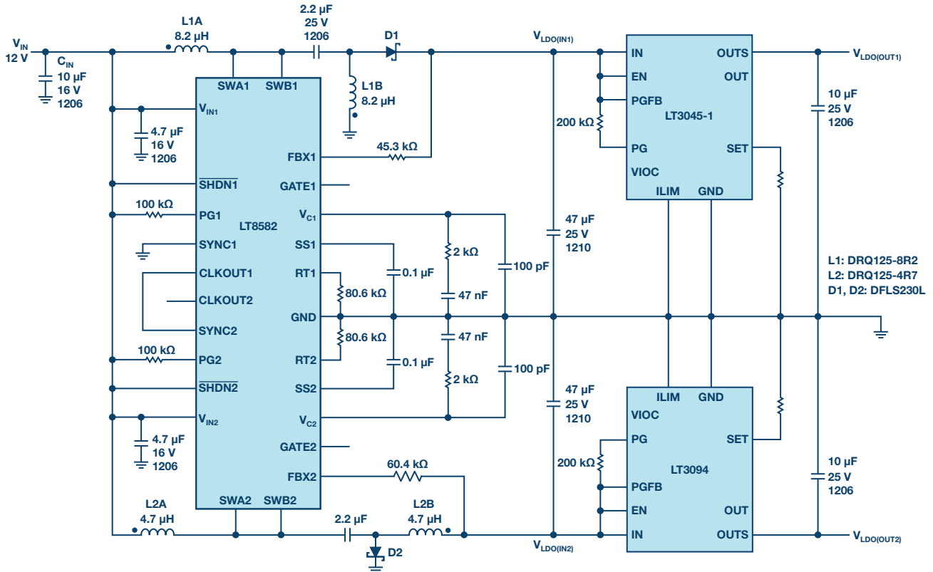
图 5. 可调节的双输出正/负电源具有高纹波抑制和低温运行性能。
