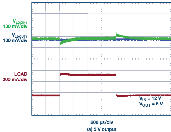
图 7.12 V 输入、 \pm 5\text{ V} 输出下的双电源瞬态响应。
