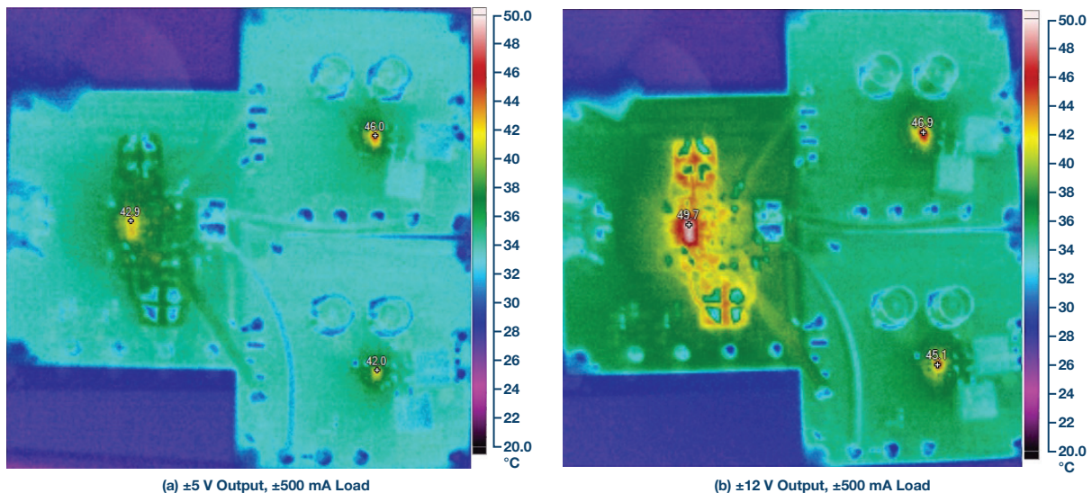
图 6. 12 V 输入下的双电源热图像。
