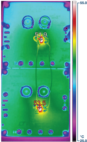
图 4. 两个并联 LT3094 的热图像。
