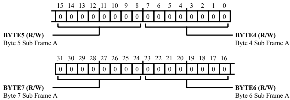
Figure 26-28: SPDIF_TX_UBUFF_A1 Register Diagram
