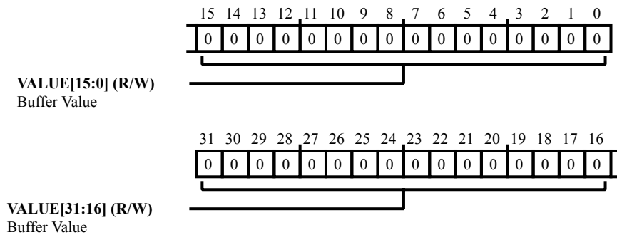
Figure 33-15: PKTE_DATAIO_BUF Register Diagram
