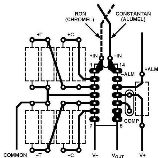
図 3. PCB 接続
