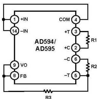
図 7. タイプ E 再キャリブレーション
