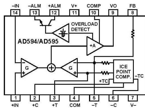
図 4. AD594/AD595 のブロック図
