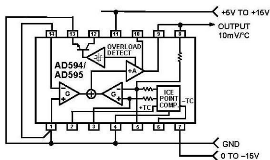
図 13. スタンドアロン摂氏温度計としての AD594/AD595
