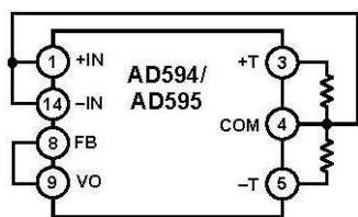
図 6. 感度減少調整
