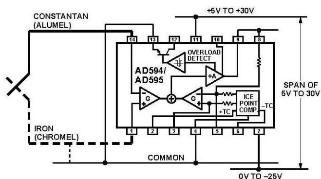
図 2. 両電源動作
