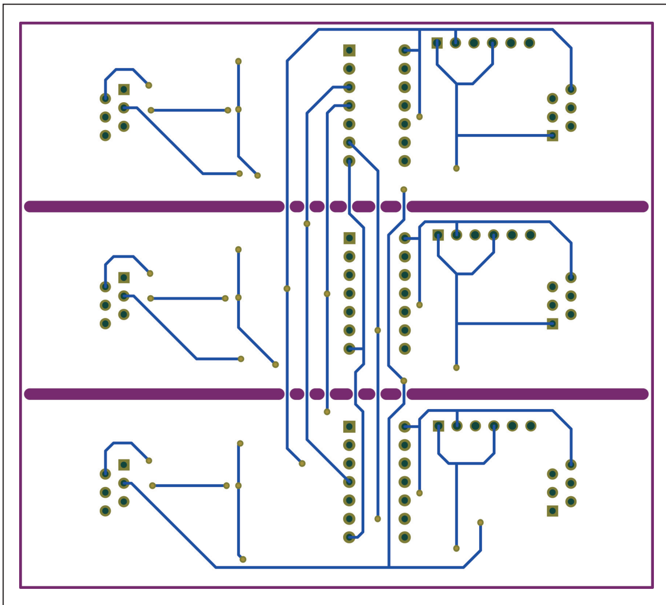
図12. EVボードのレイアウト(下面)
