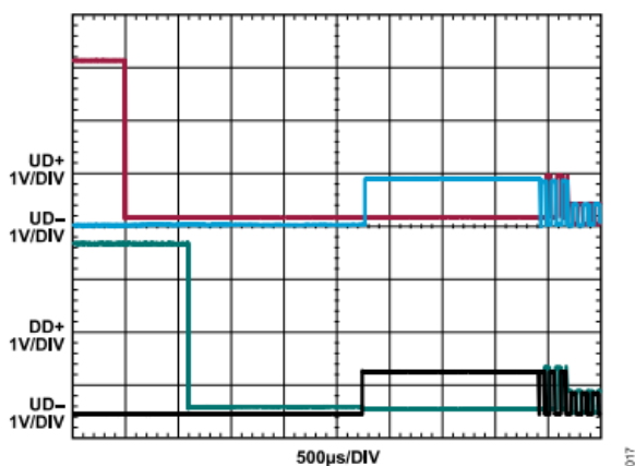
図 17. ADuM4166のハイ・スピード・ハンドシェイク
