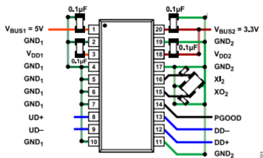
図 21. 必要な外付け部品と接続 (5V電源をサイド1、3.3V電源をサイド2に使用したADuM4166)
