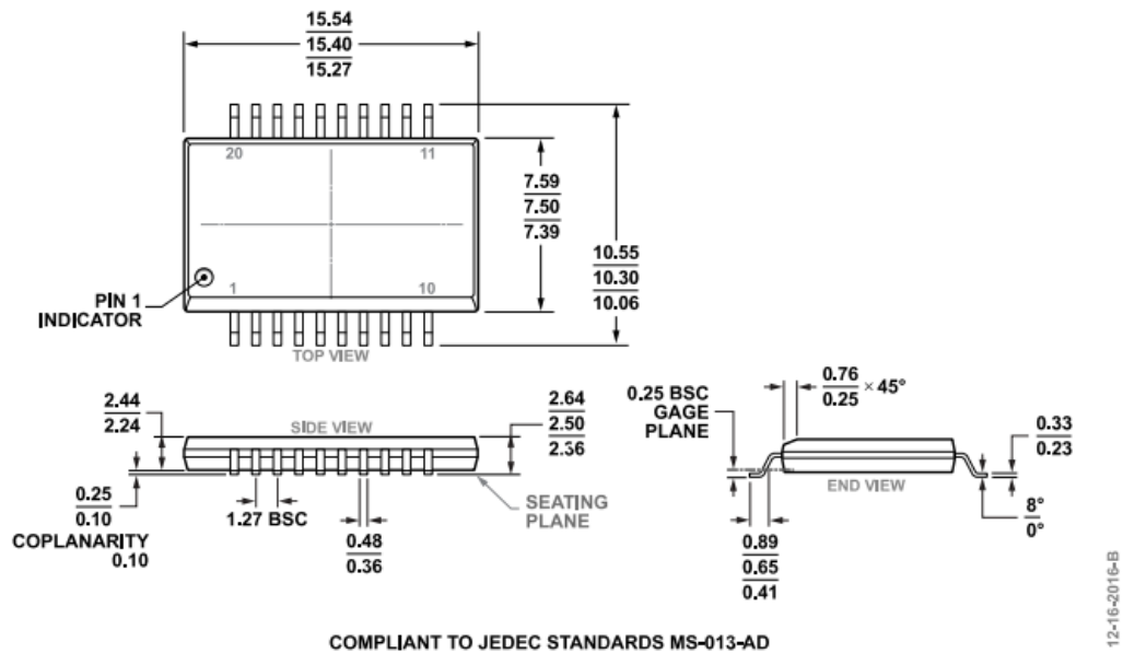
図 23. 沿面距離を増やした20ピン標準SOP（スモール・アウトライン・パッケージ） [SOIC_IC] ワイド・ボディ (RI-20-1) 寸法：mm
