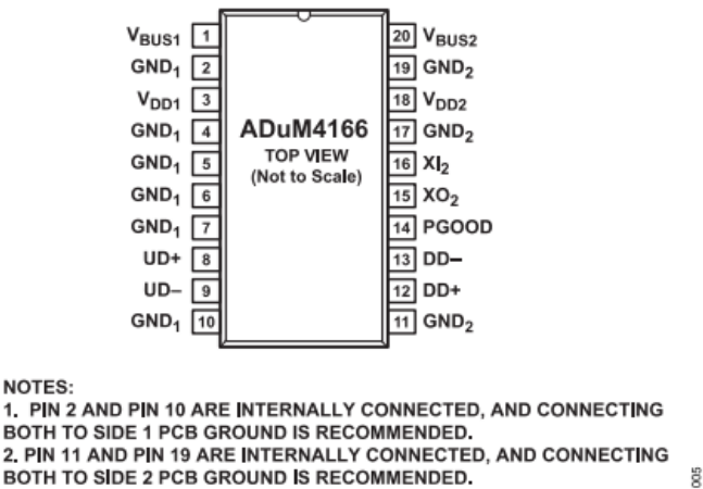
図 5. ADuM4166のピン配置
