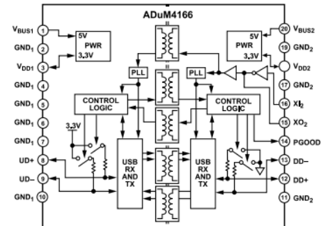
図 2. ADuM4166（ペリフェラル側からクロック入力）
