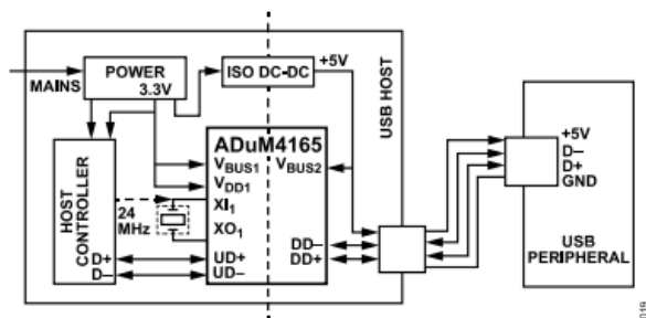
図 19. ADuM4165による絶縁型USBホスト・アプリケーション
