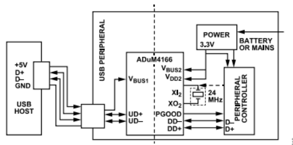
図 18. ADuM4166による絶縁型USBペリフェラル・アプリケーション
