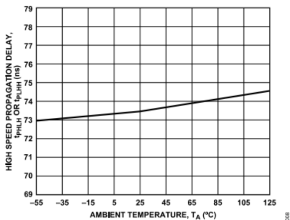
図 8. ハイ・スピードの伝搬遅延 ( t_{PHLH} または t_{PLHH} ) と周囲温度 ( T_A ) の関係
