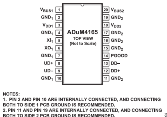
図 4. ADuM4165のピン配置
