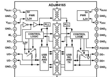
図 1. ADuM4165（ホスト側からクロック入力）
